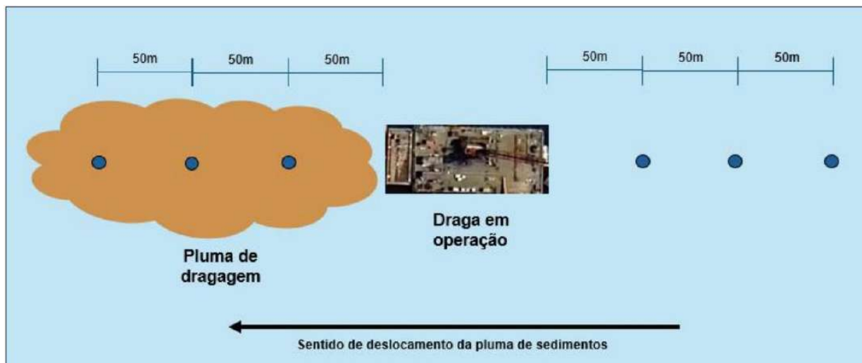
Figura 24 - Ilustração da distribuição dos pontos de amostragem de água superficial no entorno da operação da dragagem, quando a pluma de sedimentos for identificada.
