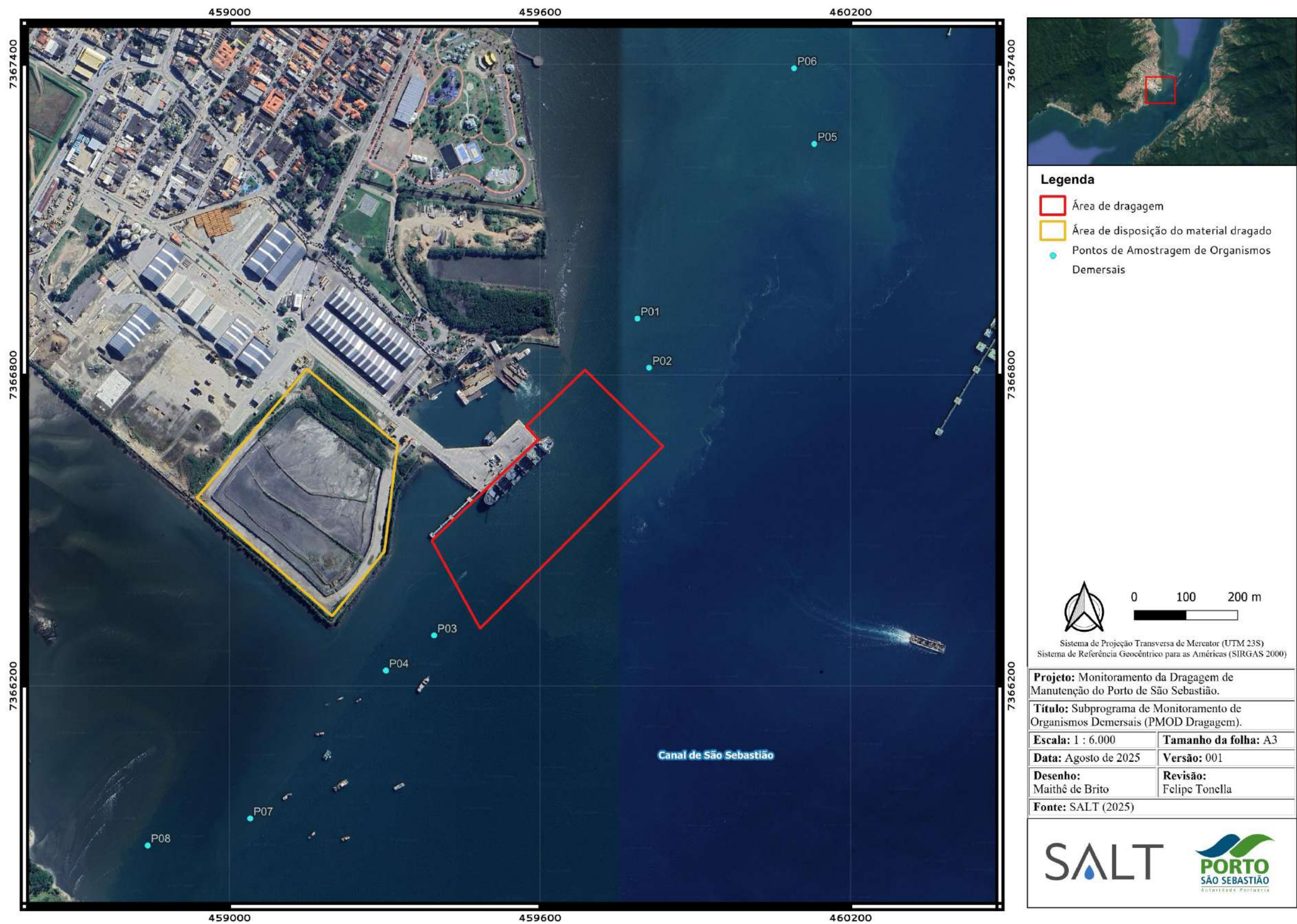
Figura 30 - Pontos de amostragem do Subprograma de Monitoramento de Organismos Demersais (PMOD Dragagem).
