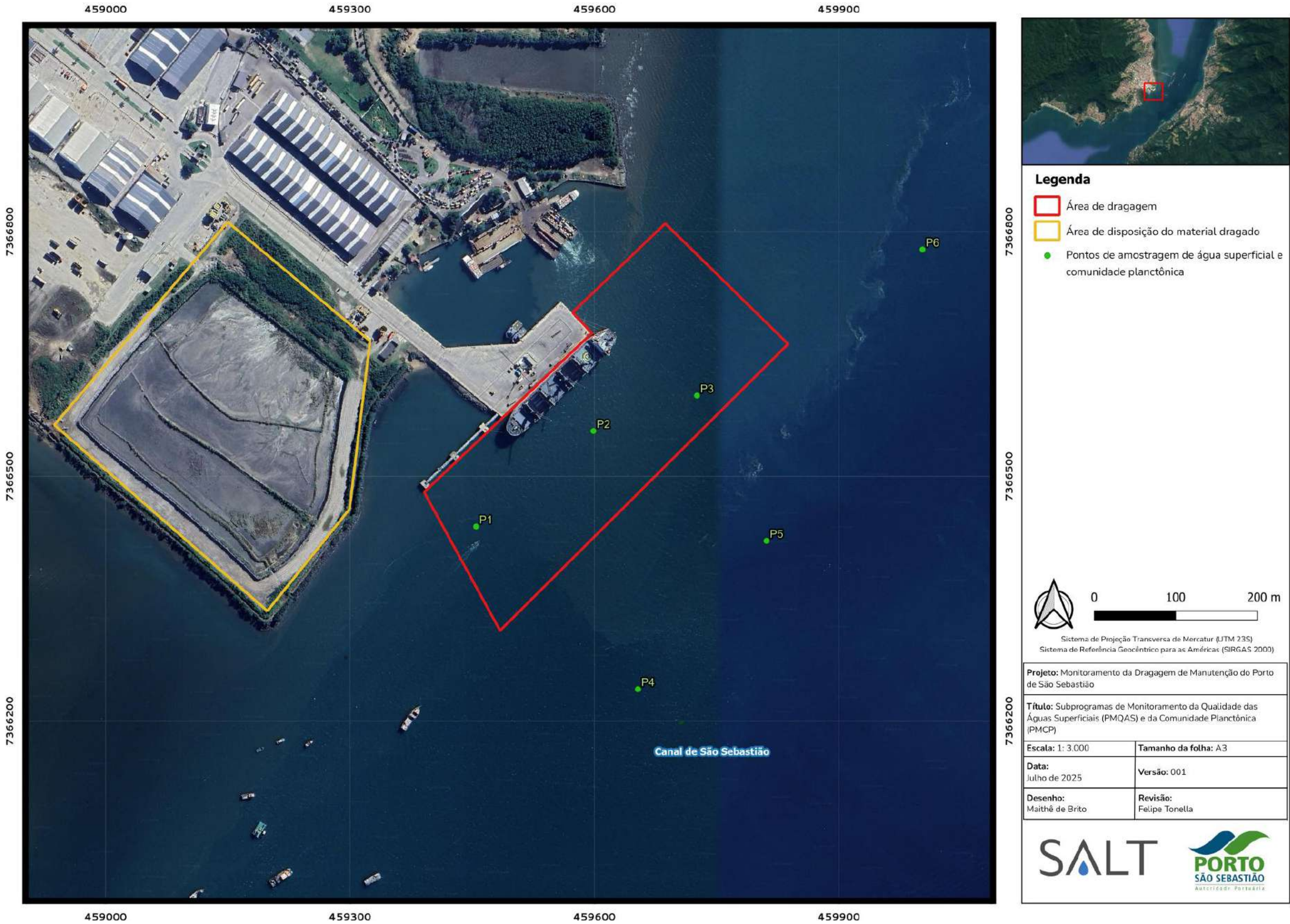
Figura 26 - Pontos de amostragem da primeira campanha do Subprograma de Monitoramento de Qualidade das Águas Superficiais (PMQAS) realizada nos dias 17 e 18 de junho de 2025.
