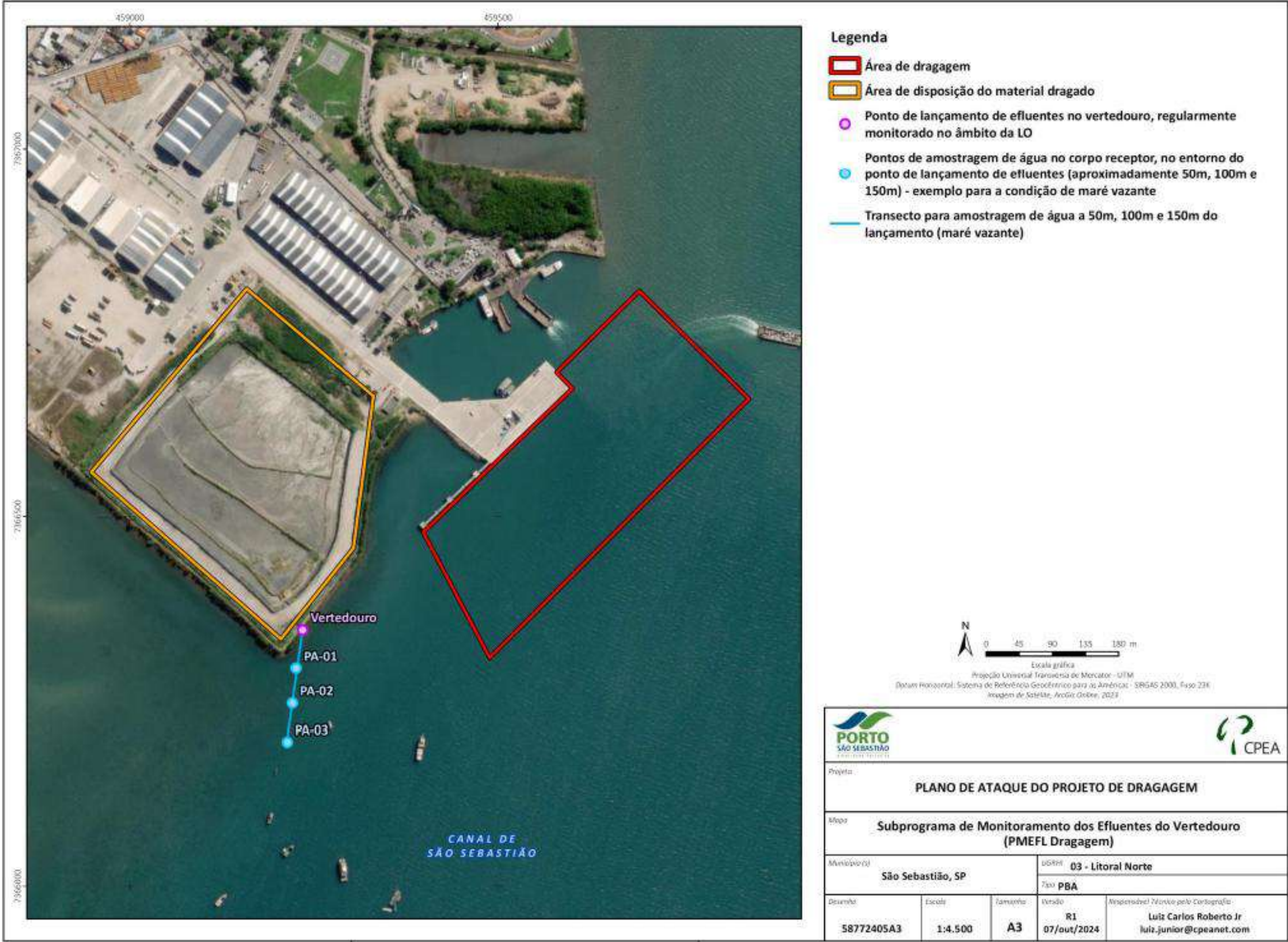
Figura 22 - Pontos de localização do Subprograma de Monitoramento dos Efluentes do Vertedouro (PMEFL) - Dragagem.
