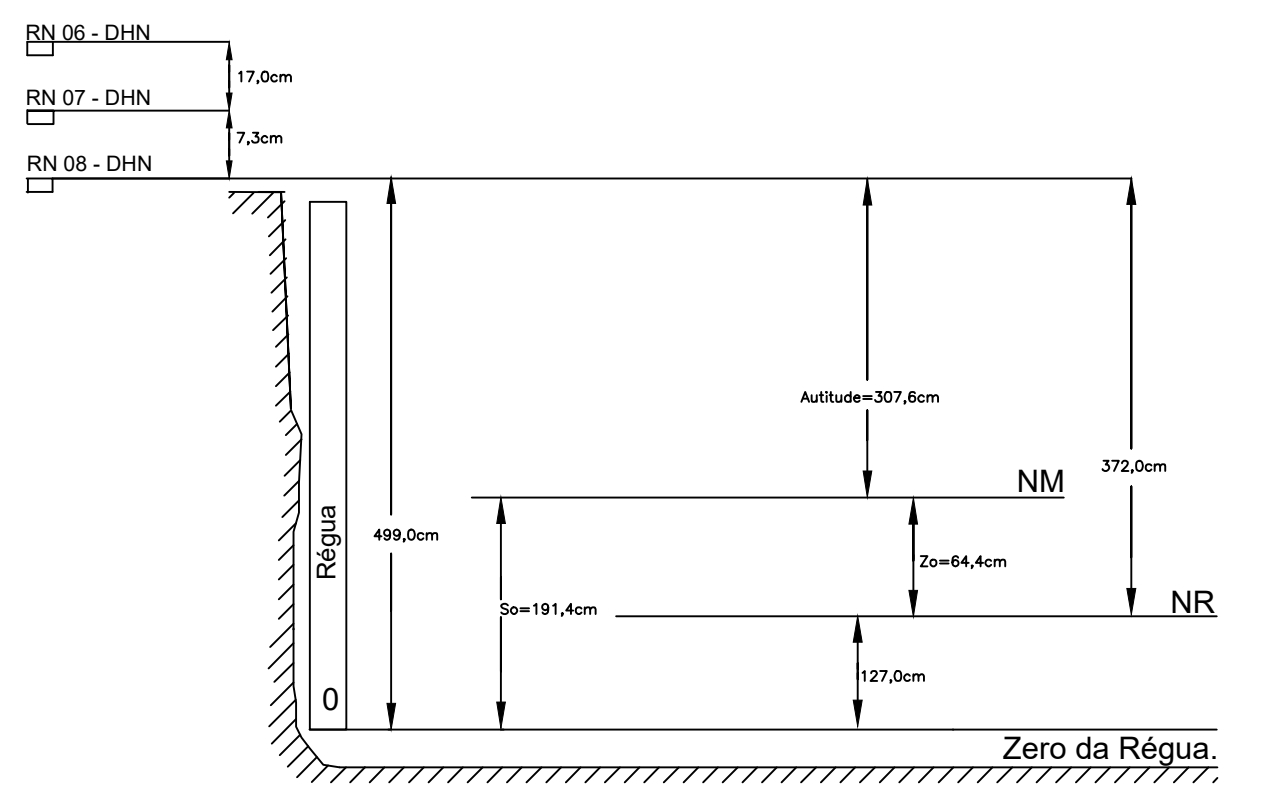
DIAGRAMA ESTAÇÃO MARÉGRAFIA PORTO DE SÃO SEBASTIÃO - F-41-1644-001/99
